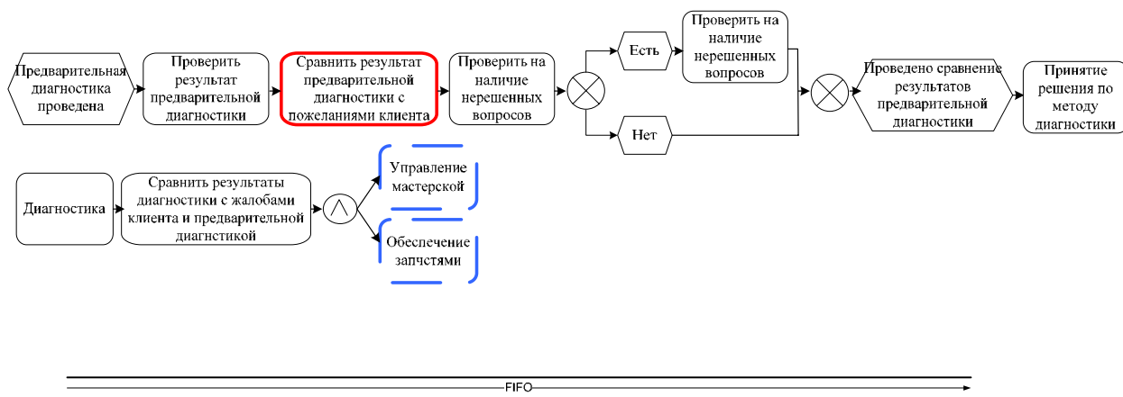
Рис. 9. Процесс «Диагностика»
